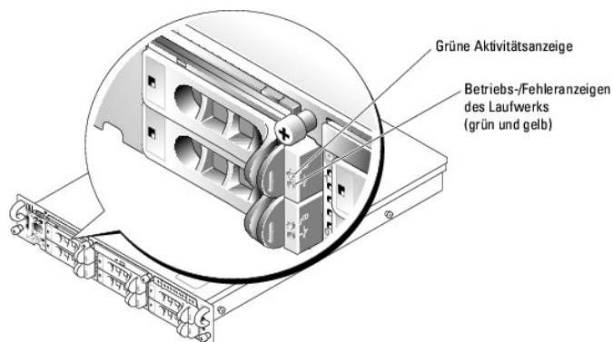
Abbildung 1-2. SCSI-Festplattenlaufwerkanzeigen
